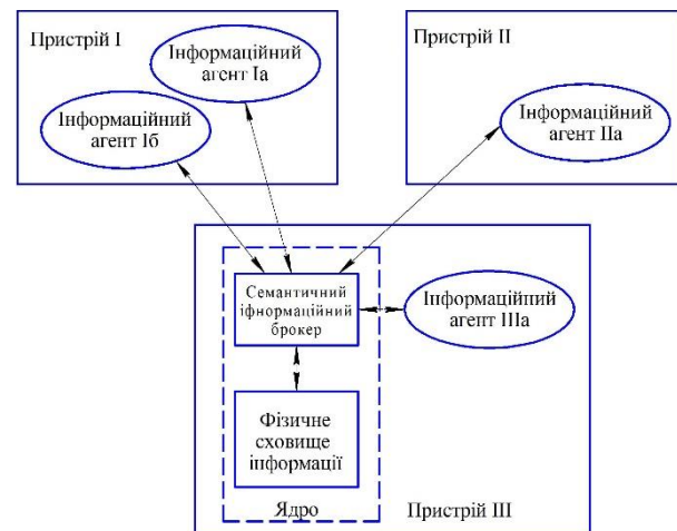
Рис. 3. Структурна схема платформи Smart-M3
