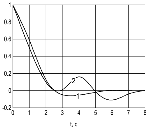
Рис. 3. Реальна (2) і апроксимована (1) нормовані кореляційні функції коливань кута повороту боронувальної ланки у поздовжньо-вертикальній площині
