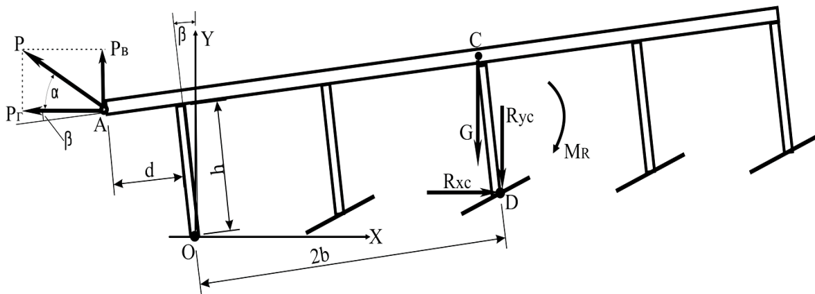
Рис. 1. Еквівалентна схема сил, які діють на боронувальну ланку під час її руху у поздовжньо-вертикальній площині
