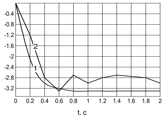
Рис. 4. Перевірка математичної моделі повороту боронувальної ланки у поздовжньо-вертикальній площині на адекватність: 1 – теоретична залежність; 2 – експериментальна залежність
